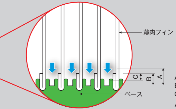
Jフィン カシメ部の拡大図
